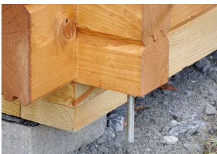
Gewindestangen ab Wandstärke 44 mm
