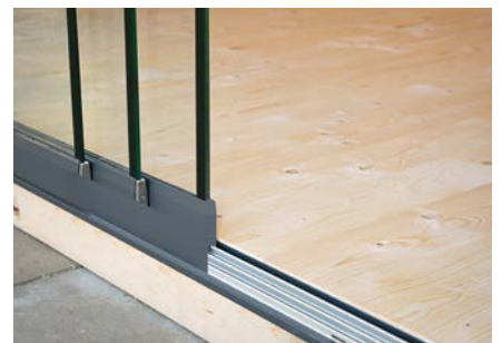
Schiebetür für Alvina
